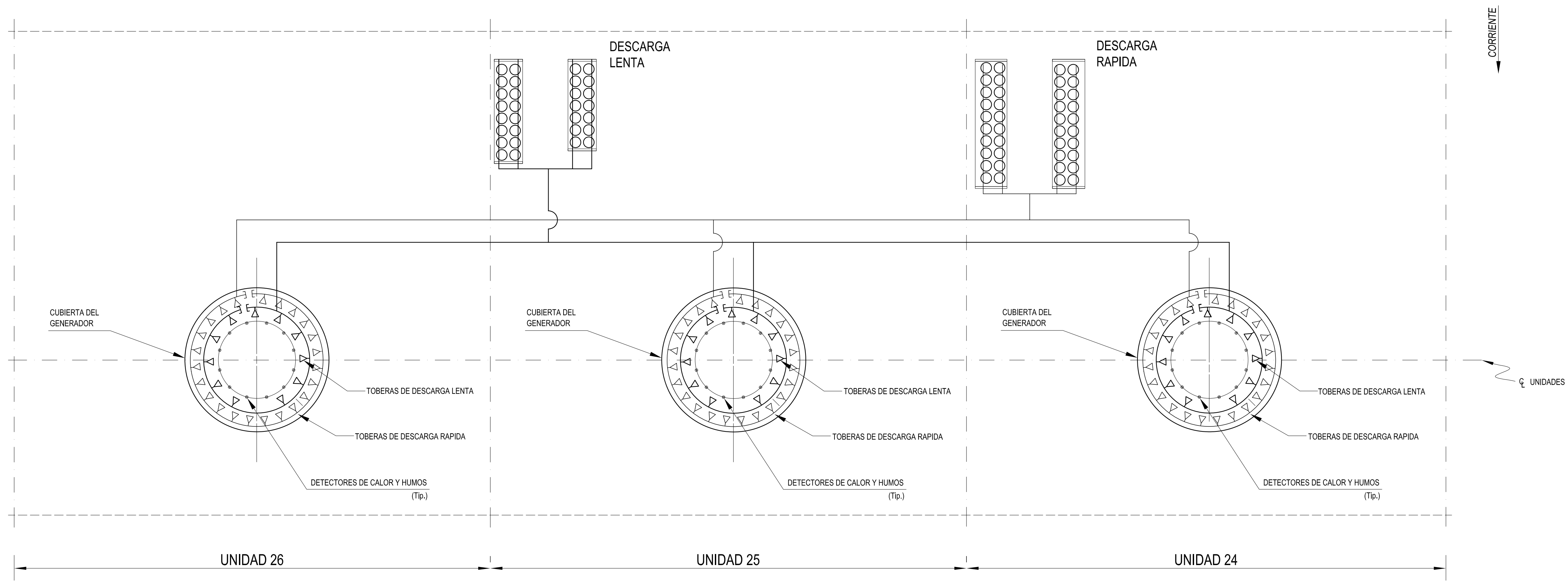
SISTEMA DE CO 2 DE PROTECCION CONTRA INCENDIOS PARA GENERADORES
